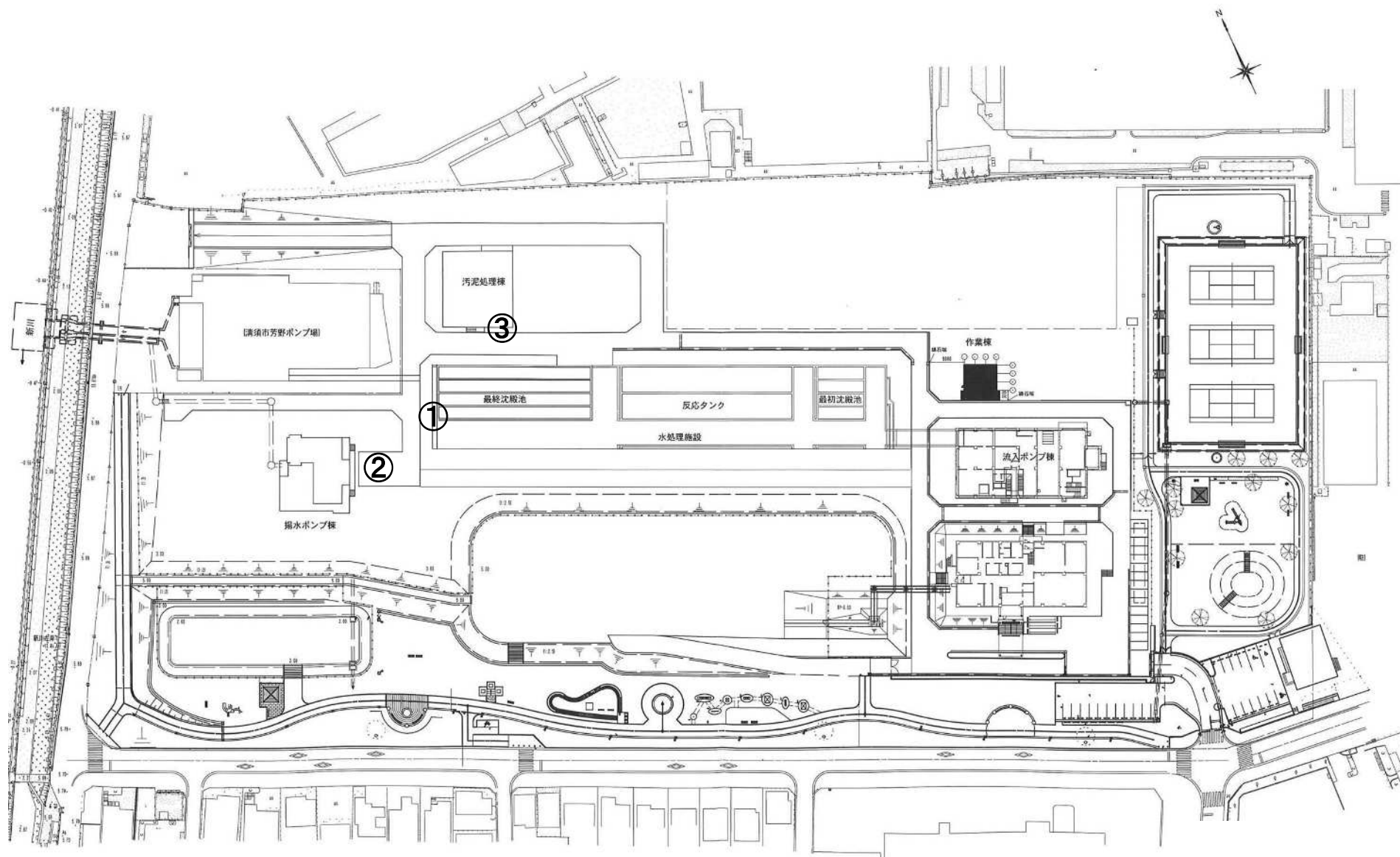
新川西部浄化センター 場内平面図
