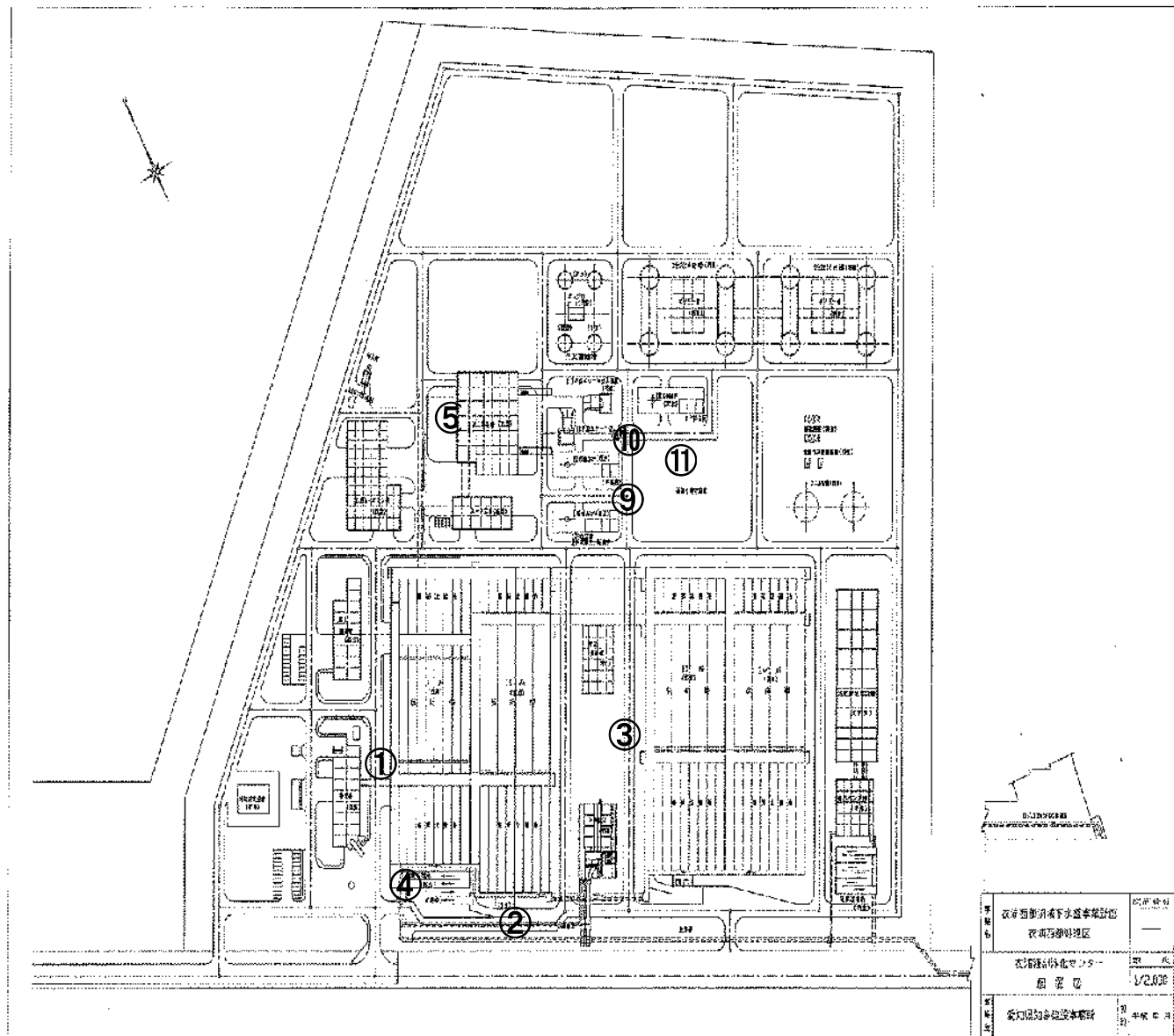
衣浦西部浄化センター場内平面図
