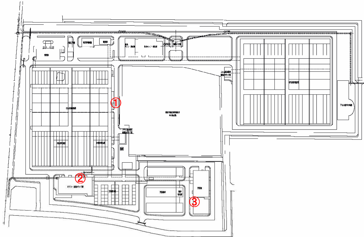
日光川上流浄化センター全体配置図
